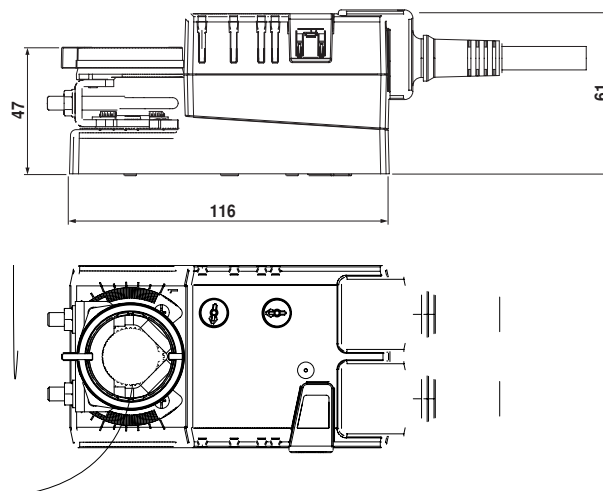
Rozměrové schéma
