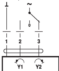
Schémata zapojení AC 24 V, 3bodové
