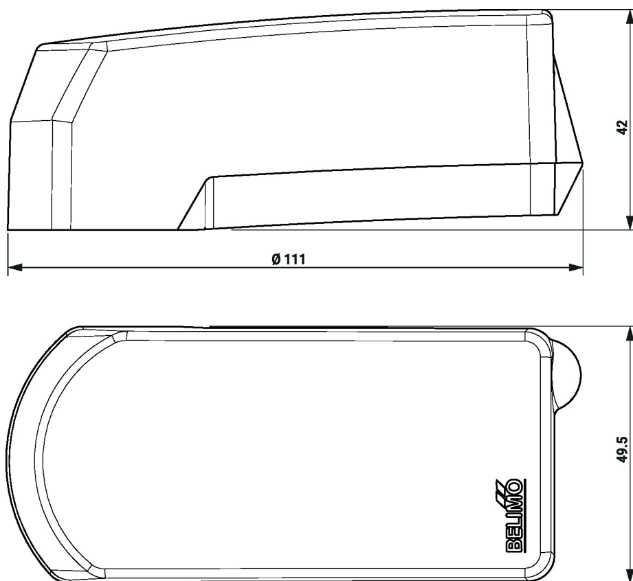
Rozměrové schéma
